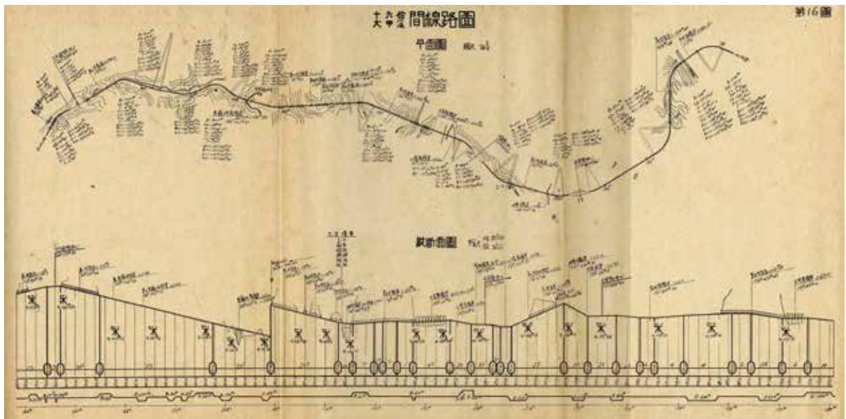
從舊山線地形剖面圖可見此路段工程的艱難 (苗栗縣政府文化觀光局建檔, 發佈於國家文化記憶庫。)
