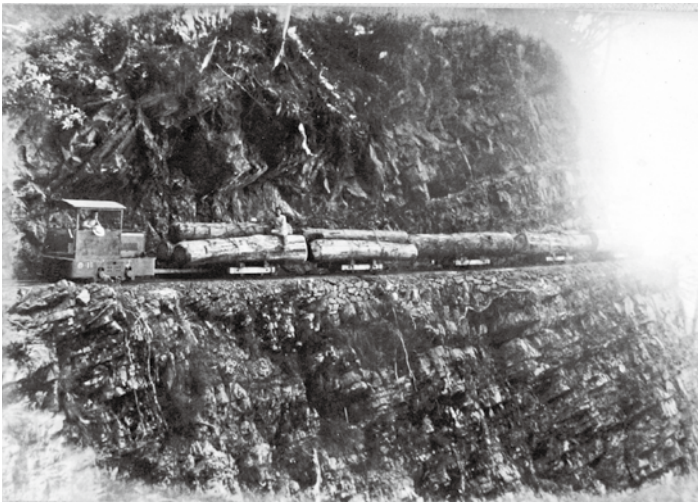
八仙山的運材機關車可以加掛車廂兼營載客
