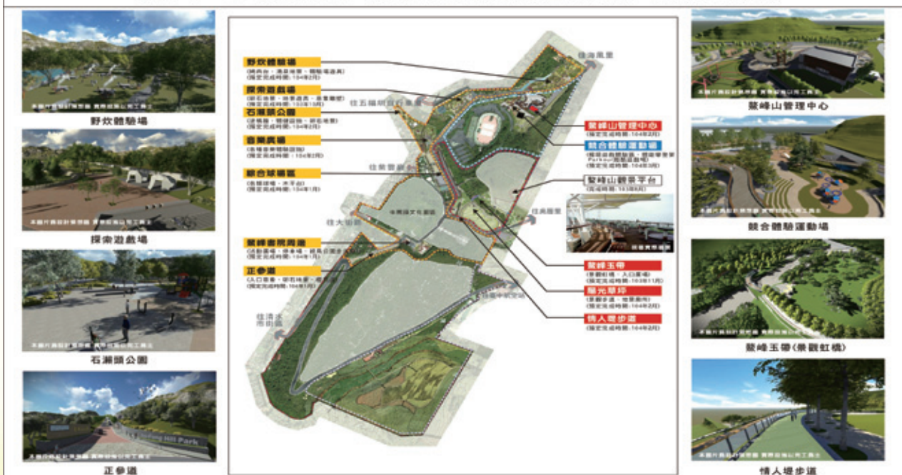
▲鰲峰山公園整體發展建設全區工程配置圖
